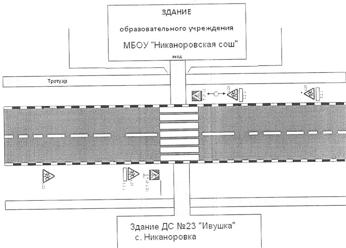
Схема организации дорожного движения вблизи МБОУ "Никаноровская сош"
